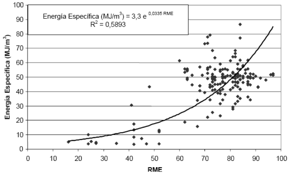
Figura 5. Correlación entre el RME y la Energía Específica.
