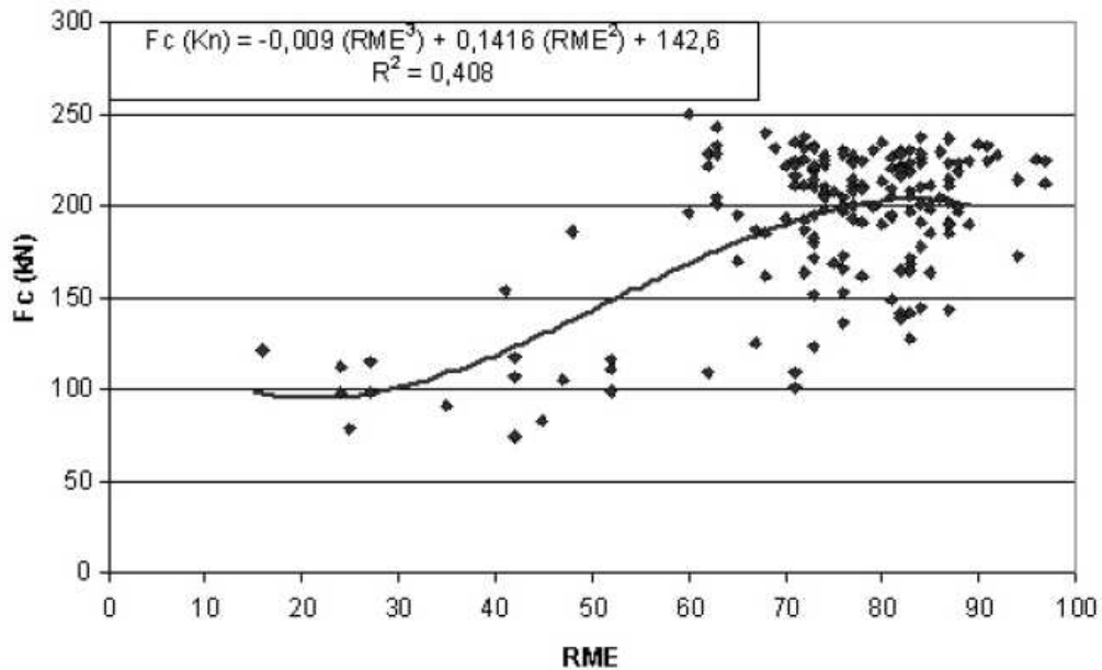
Figura 8. Correlación entre el RME y el empuje por cortador aplicado en la cabeza de corte.
