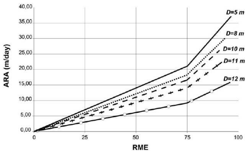
Figura 4. Correlación entre ARA (m/día) y RME para distintos diámetros de excavación.
