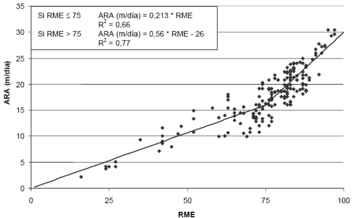
Figura 3. Correlación entre ARA (m/día) y RME.
