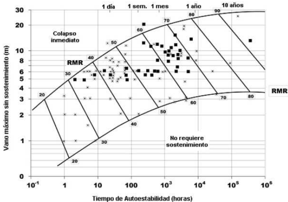
Figura 2. Tiempo de autoestabilidad en función del RMR y de la máxima distancia sin sostenimiento.
