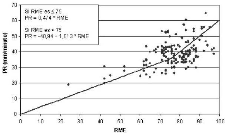
Figura 6. Correlación entre el RME y la Penetración Neta.
