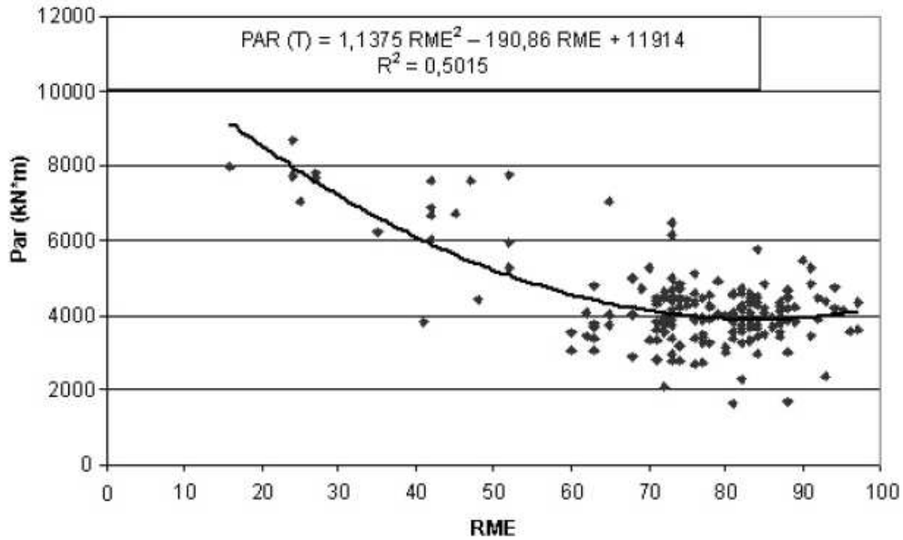
Figura 7. Correlación entre el RME y el par (T) aplicado en la cabeza de corte.
